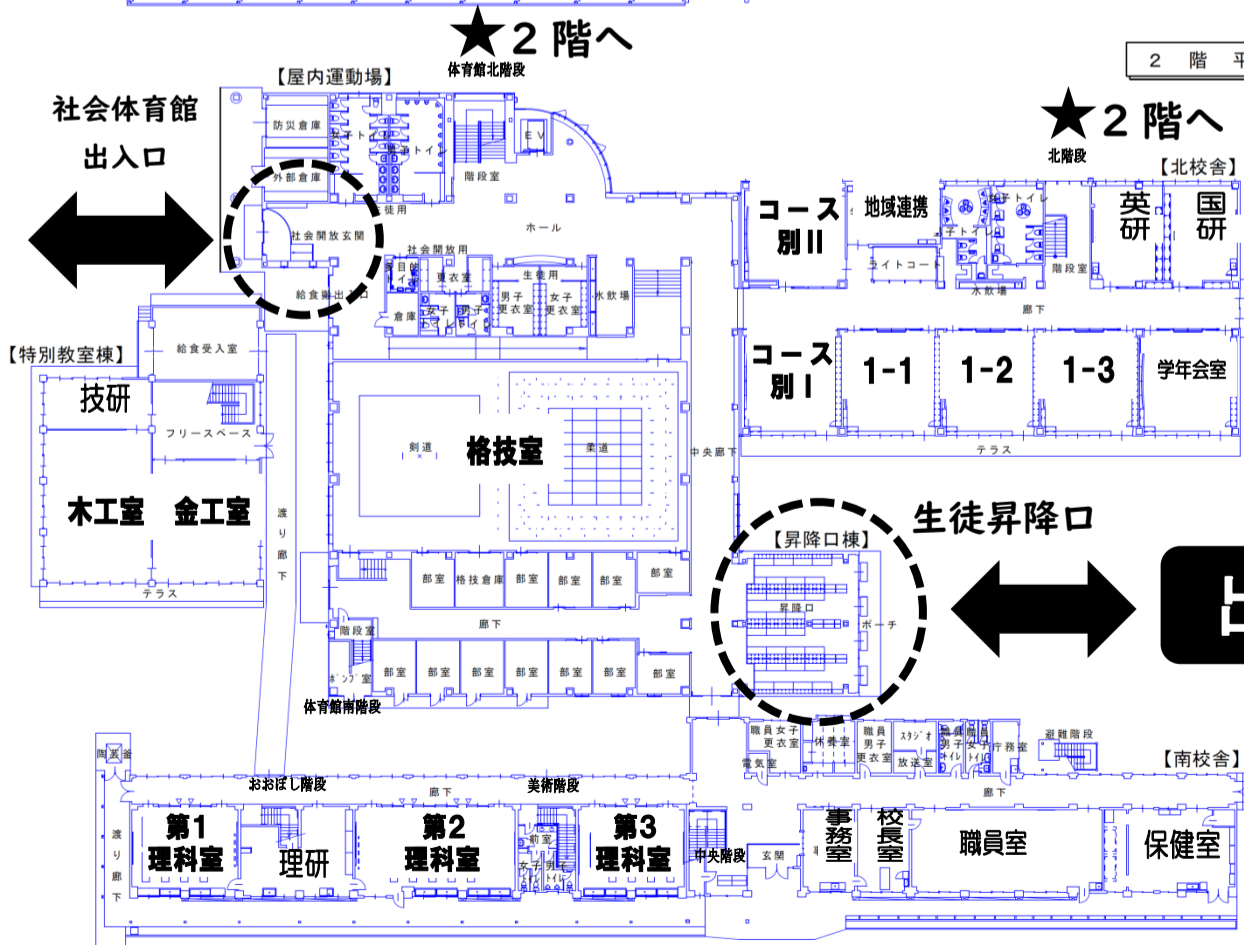
1階平面図
